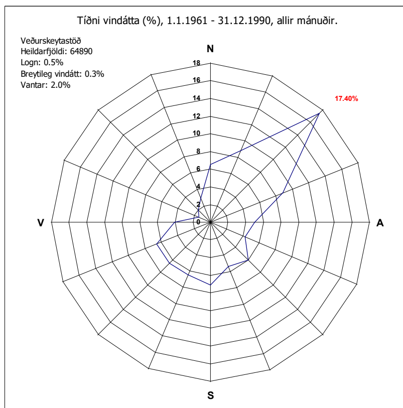
MYND 4.23 Tíðni vindátta á Eyrarbakka samkvæmt 30 ára meðaltali árána 1961-1990.
