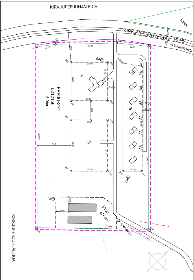
AFSTÖÐUMYND m.kv 1:1.000
