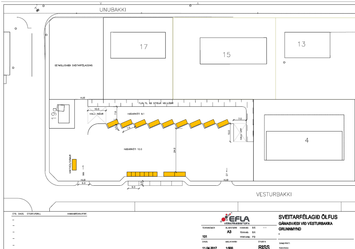
Mynd 2. Líklegt fyrirkomulag á gámasvæði við Vesturbakka í Þorlákshöfn.
